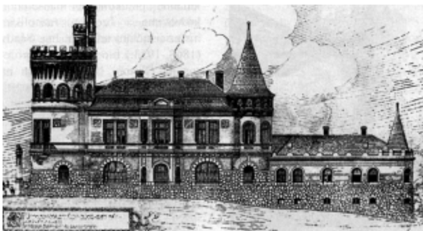
Autorski crtež sjevernog pročelja
