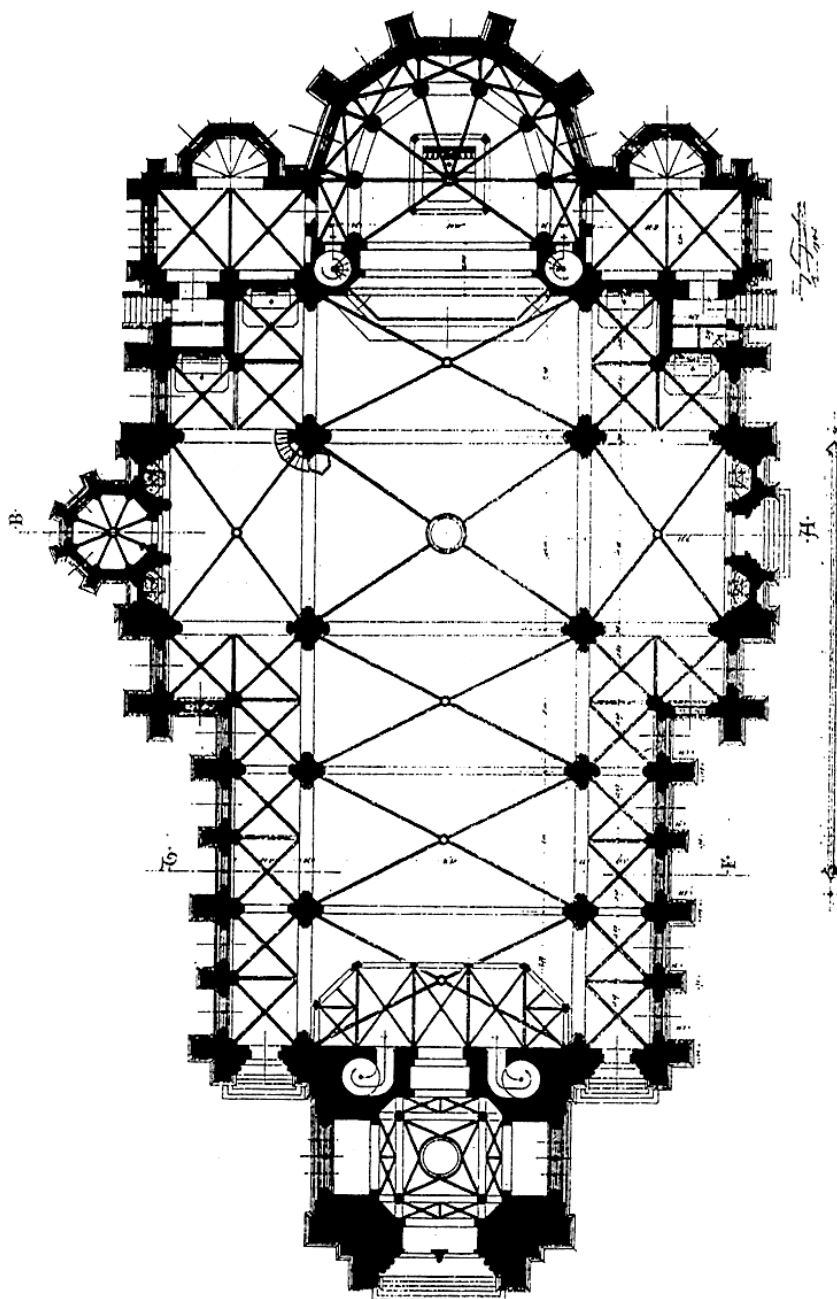
Tlocrt.
