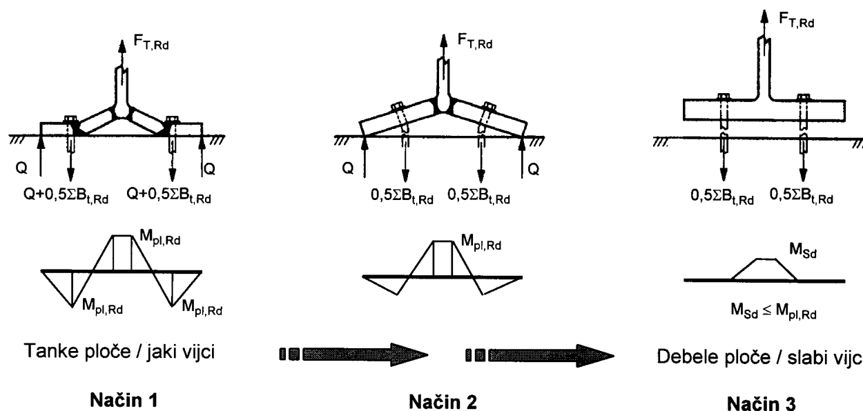
Slika 3. Načini otkazivanja pojasnice T-komada
