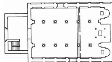
Tlocrt ranoromaničke krunidbene bazilike Sv. Petra i Mojsije
