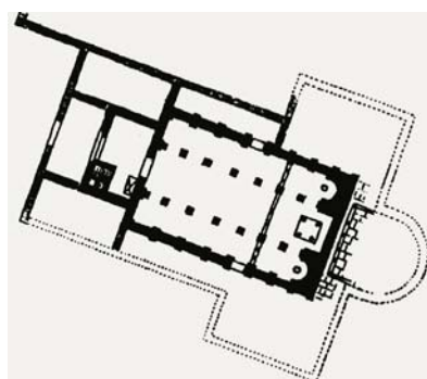
Prvi tlocrt ranokršćanske i ranoromaničke crkve Sv. Petra i Mojsije
