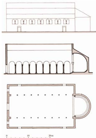
Pogled, presjek i tlocrt starokršćanske crkve
