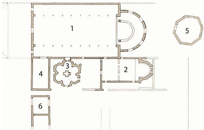
Rekonstrukcija tlocrta episkopalnog kompleksa krajem 4. i početkom 5. st.: 1. bazilika, 2. katekumenej (sada sakristija), 3. krstionica, 4. dijakonikom, 5. oktogon, 6. episkopij
