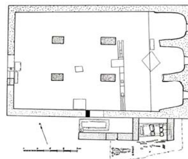
Tlocrt grobljanske bazilike Sv. Šimuna u Guranu (prijašnja istraživanja)
