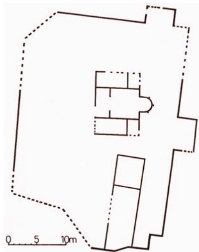
Tlocrt bizantske utvrde i crkve na Gradini na otočiću Osinju
