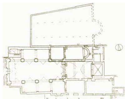
Pretpostavljeni tlocrt starokršćanske katedrale (gore) uz sadašnju hvarsku katedralu
