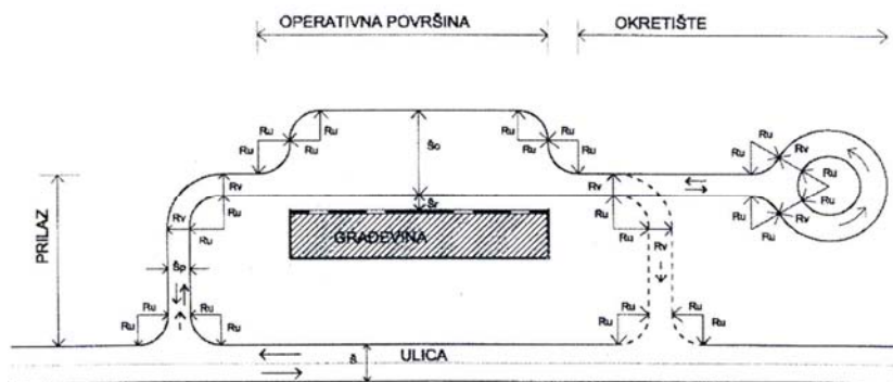
Slika 6. Horizontalna shema vatrogasnog pristupa
