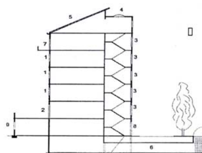
1 prozor 2 terasa 3 ostakljeno stubište 4 i 5 otvori i pokrov krova 6 podzemni sig. ulaz 7 balkon 8 ulazna vrata 9 montažni otvor na zidu
