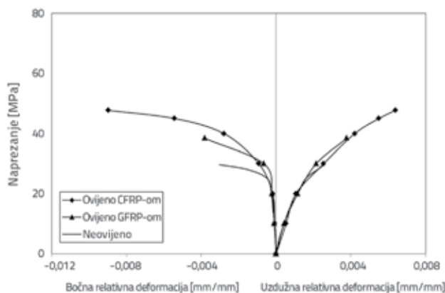
Slika 4. Odnos naprezanje–relativna deformacija ovijenog i neovijenog betona čvrstoće 30 MPa
