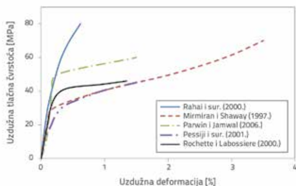
Slika 1. Odnos naprezanje – relativna deformacija različitih ovijenih uzoraka
