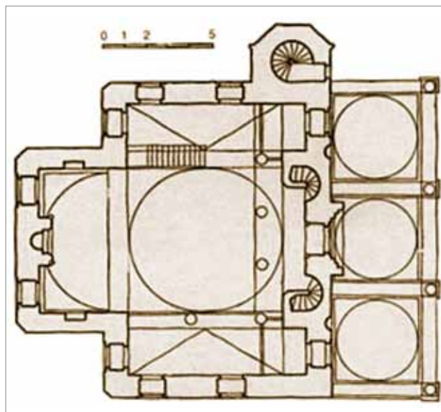
Tlocrt džamije
