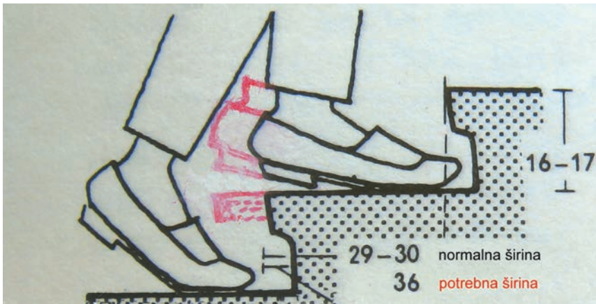
Skica gazišta na stubištima koja su manja od dužine cipela
